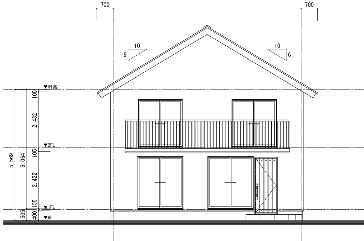
南側立面図
