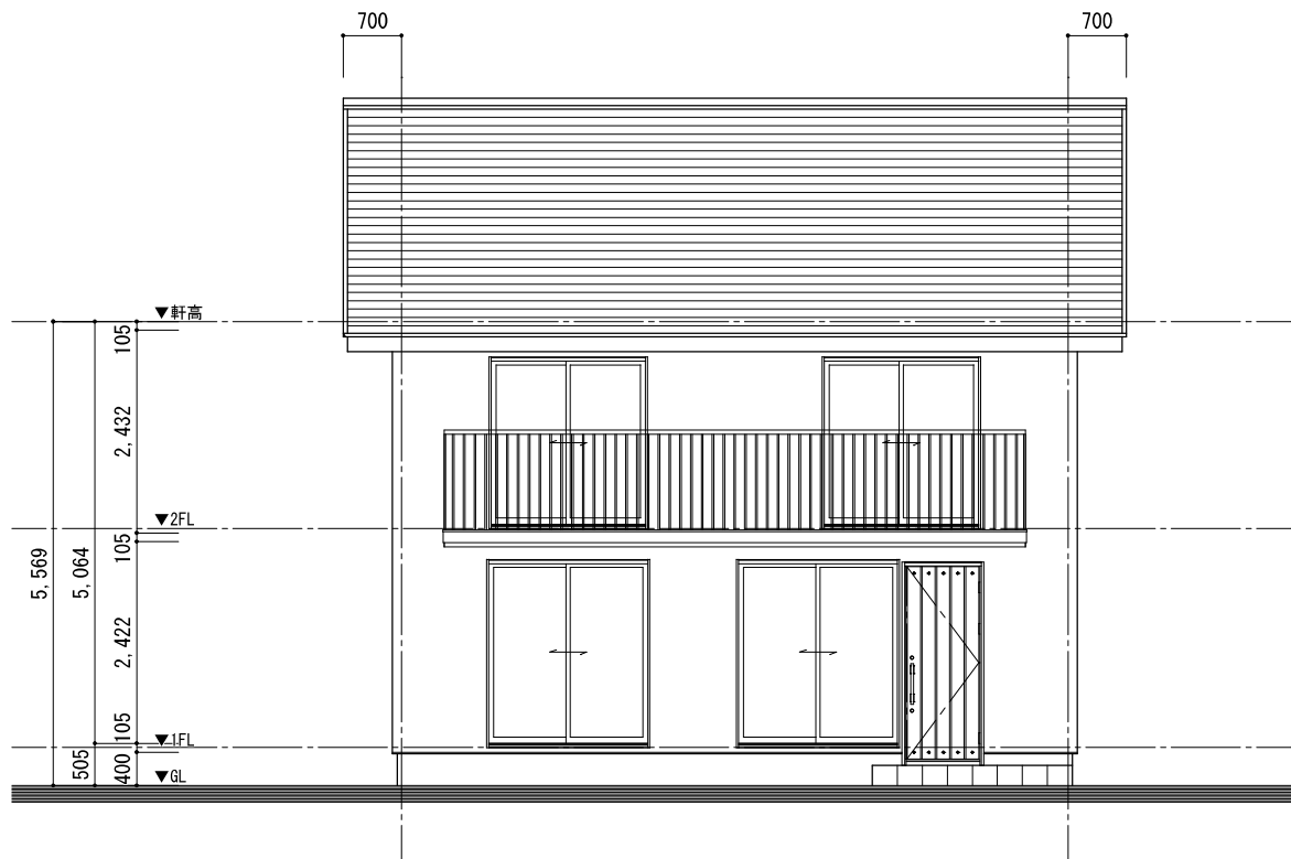
南側立面図
